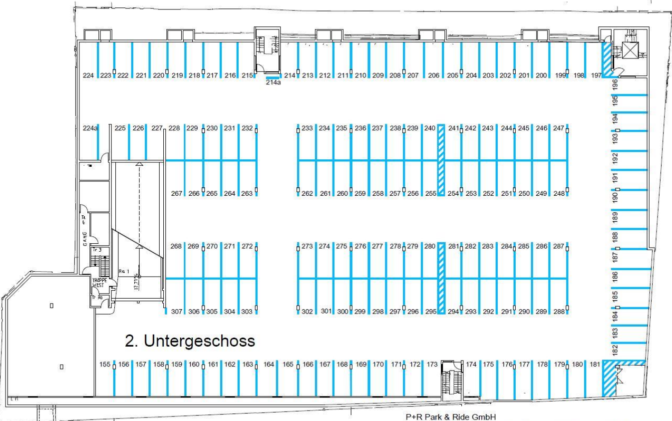
P+R Park & Ride GmbH Anwohnergarage Kellerstraße, Stellplatzmarkierung und -Nummerierung 2. Untergeschoss, o. Maßstab / 23.03.2017 / Weigl
